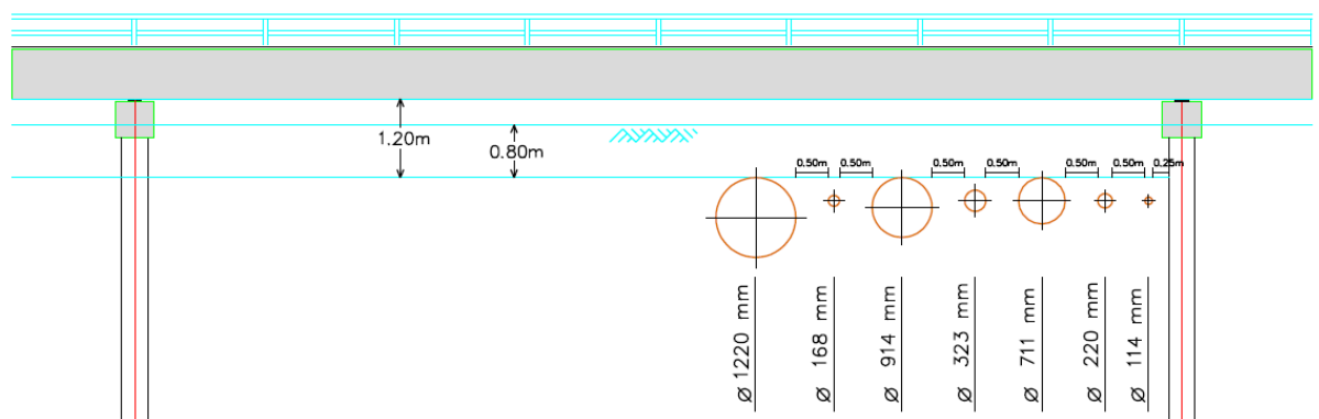
Figuur 3 – Leidingen onder viaduct
