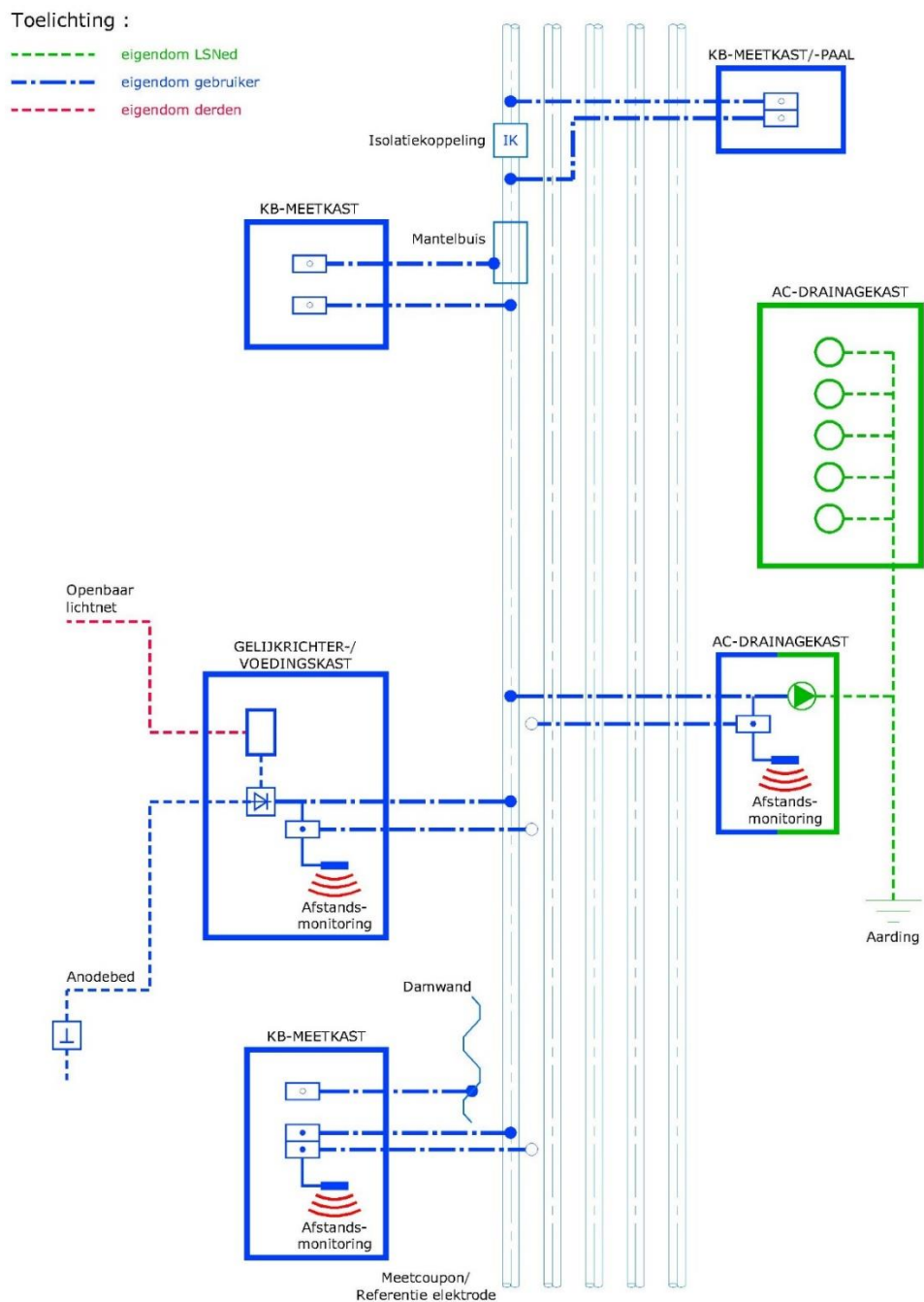
Figuur 5 – Principe eigendomsafbakening eigen KB-systeem
