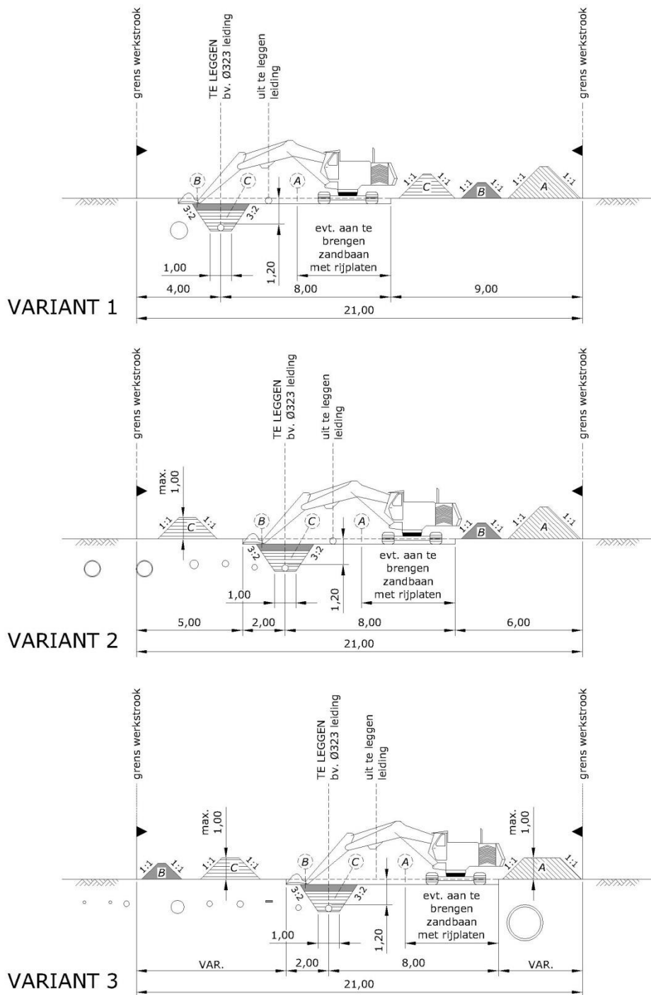
Figuur B.1 – Principevoorbeelden werkstrookindeling
