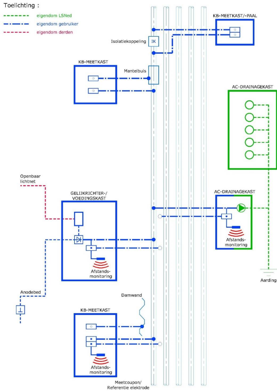
Figuur 3 – Principe eigendomsafbakening eigen KB-systeem
