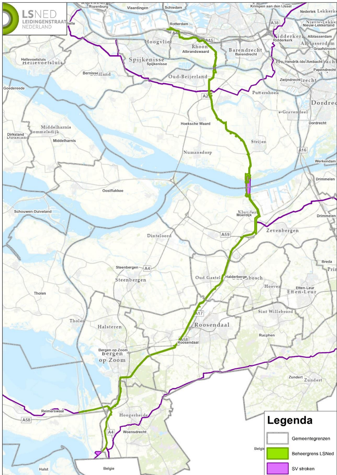
Figuur 1 – Het tracé van de Buisleidingenstraat en de aansluitende leidingstroken uit de Structuurvisie Buisleidingen 2012-2035
