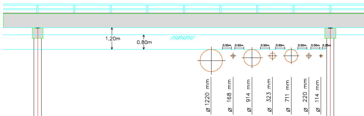
Figuur 3 – Leidingen onder viaduct
