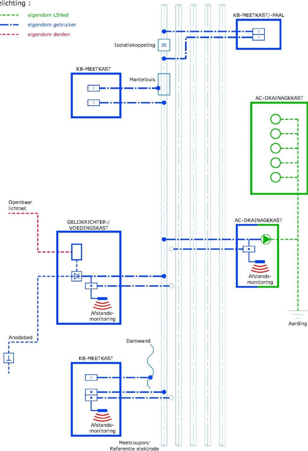
Figuur 5 – Principe eigendomsafbakening eigen KB-systeem
