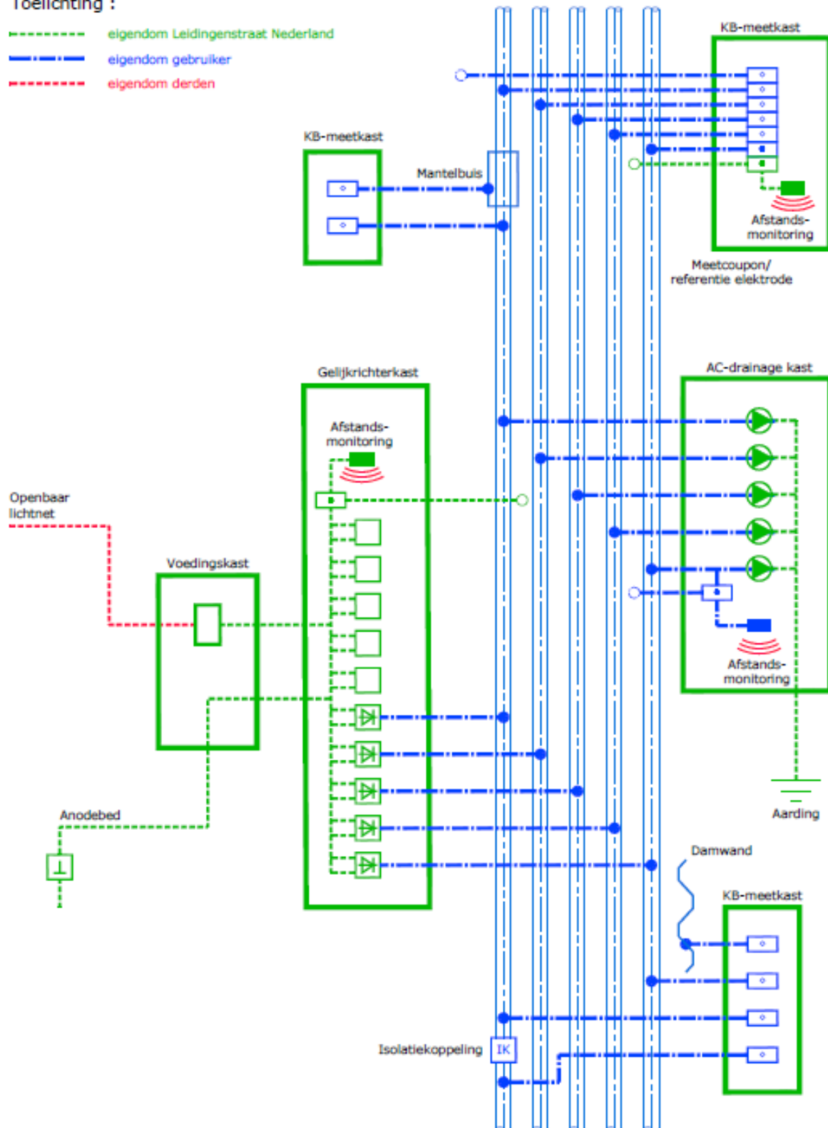
Figuur 4 – Principe eigendomsafbakening gezamenlijk KB-systeem LSNed
